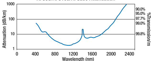
AFS50/AFS105/AFS200 Attenuation
